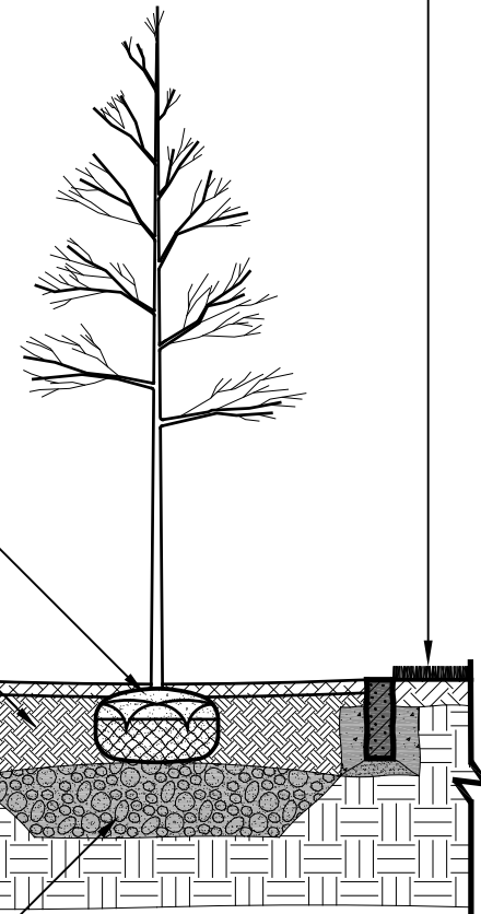
SECTION A-A
